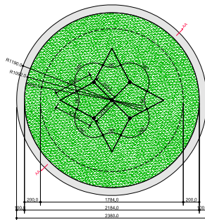
Pianta Scala 1:100 Dimensioni in cm
