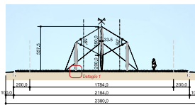
Sezione A-A Scala 1:100 Dimensioni in cm
