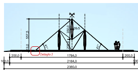
Sezione A-A Scala 1:100 Dimensioni in cm
