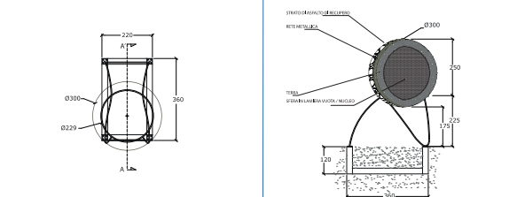
PROSPETTO FRONTE/RETRO PLANIMETRIA PROSPETTO LONGITUDINALE SEZIONE A - A'
